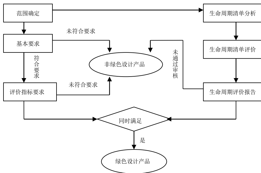
图 1 二氧化硫绿色设计产品评价流程
