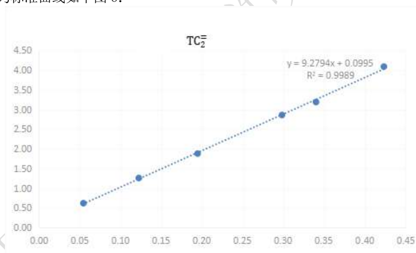
图 6：榆林化工公司建立的无规共聚聚丙烯乙烯含量标准曲线
