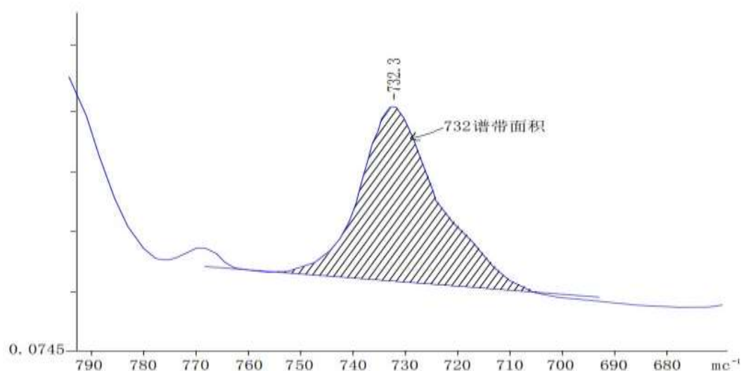
图1 无规共聚聚丙烯中亚甲基链谱带峰面积
