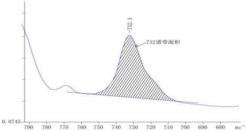
图1 无规共聚聚丙烯中亚甲基链谱带峰面积
