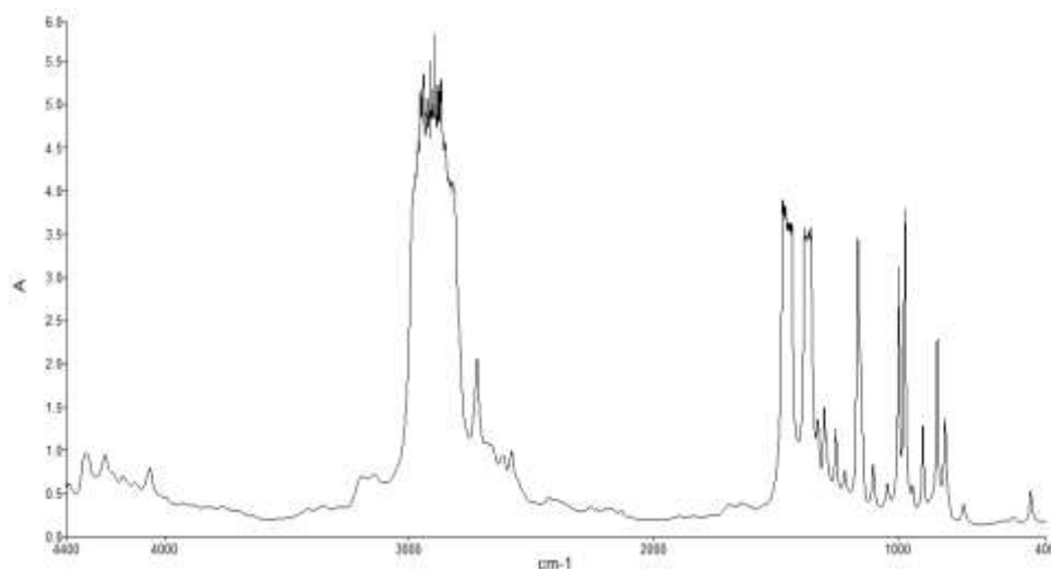
图 3: INEOS 工艺榆林化工公司 T4401 无规共聚聚丙烯典型谱
