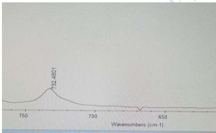
图 4: UNIPOL 工艺包头化工公司 MT35 无规共聚聚丙烯典型谱图
