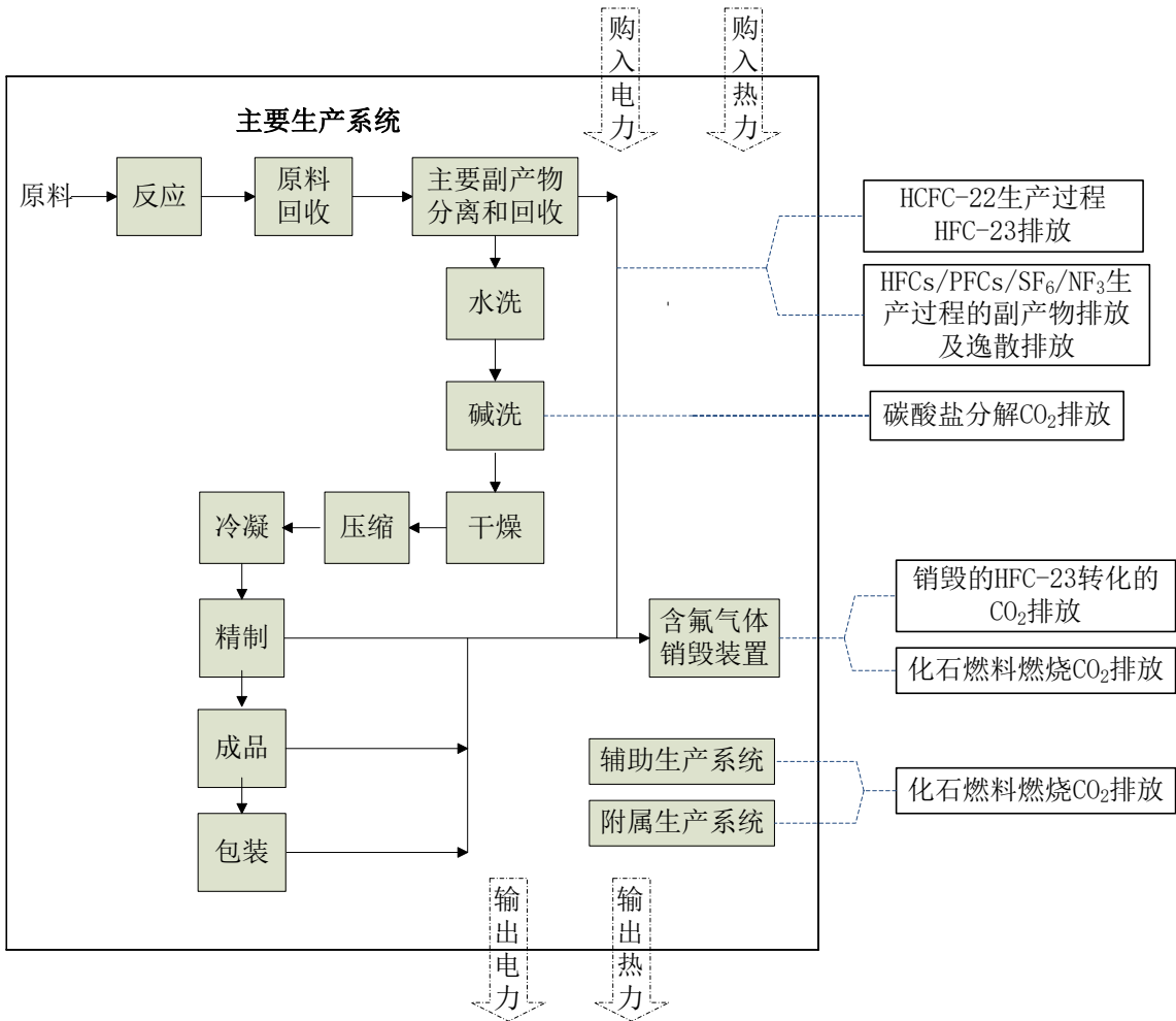
图A.1 氟化工企业碳排放核算边界示意图
