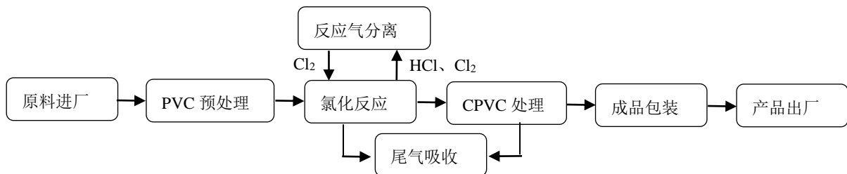
图 B.1 气固相相法氯化聚氯乙烯树脂产品生命周期系统边界图
