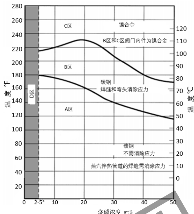
图 B.5.1 碳钢在烧碱溶液中的应力腐蚀
